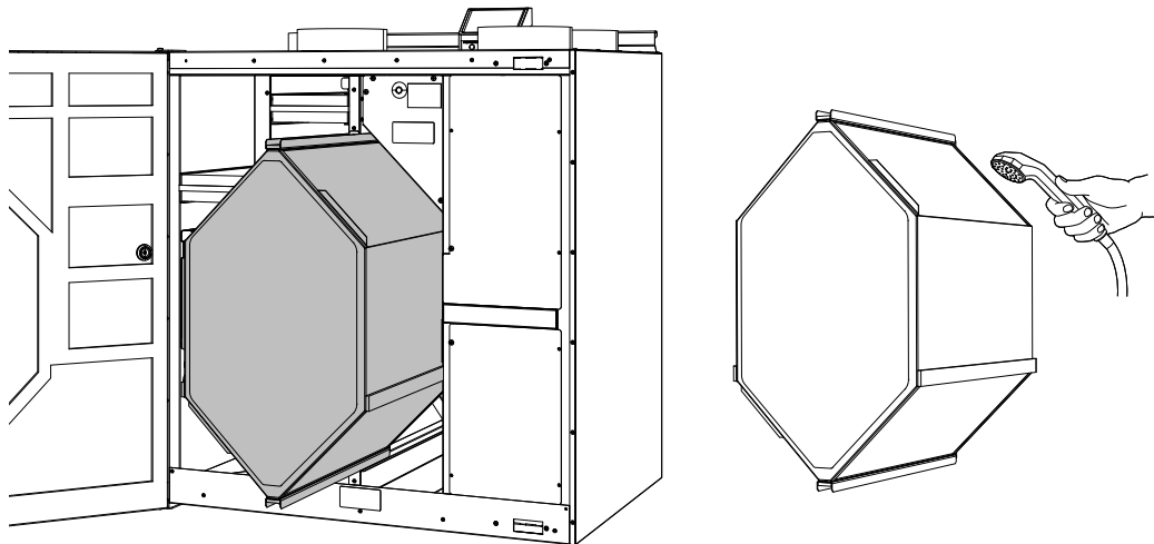
Obr. 5 Vybratie a čistenie výmenníka tepla
