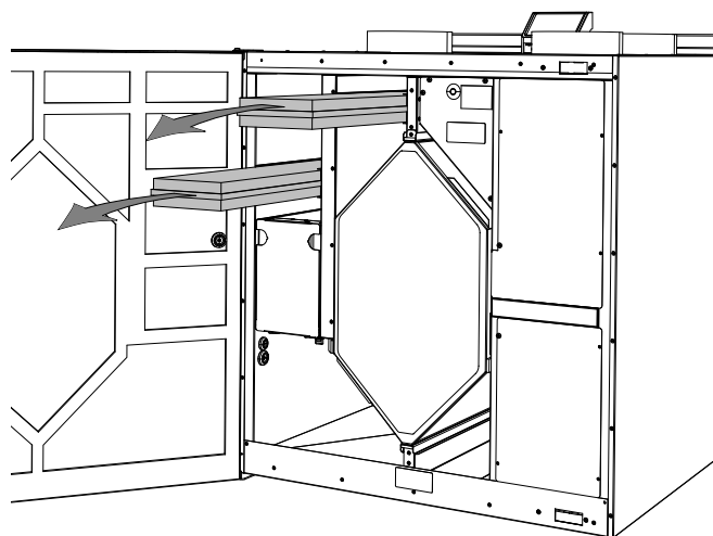
Obr. 4 Výmena filtrov
