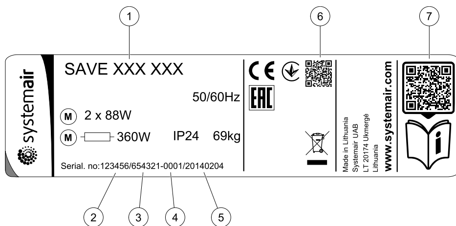
Obr. 1 Typový štítok
