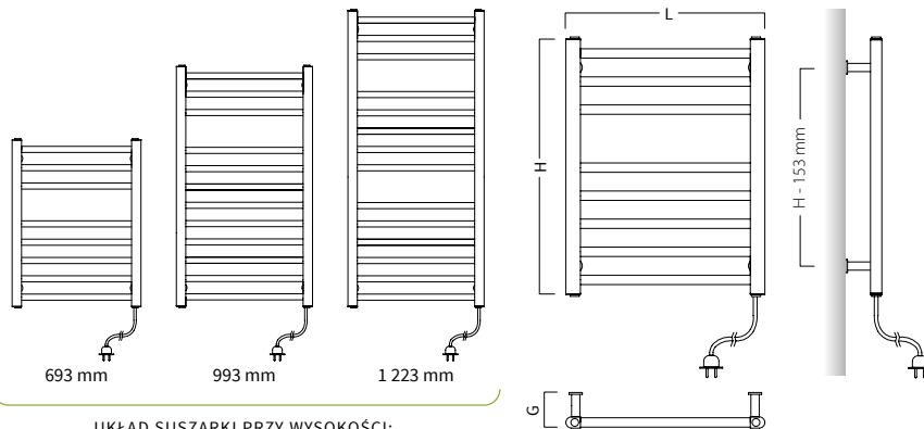
UKŁAD SUSZARKI PRZY WYSOKOŚCI: towel rail shape and design with the height:
