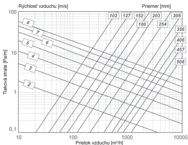
Graf : Tlaková strata v závislosti na prietoku vzduchu
