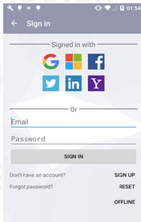
Obrázok 13: Prihlasovacia obrazovka
