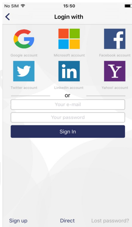
Obrázok 1. Prihlasovacia obrazovka
