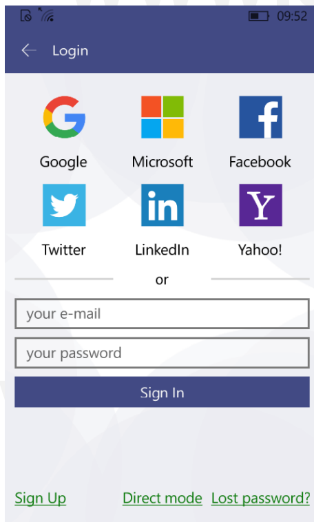
Obrázok 26. Prihlasovacia obrazovka
